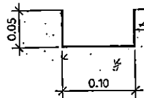
แบบขยายวางระบายน้ำแผ่นสแลตด้วย 1 : 5
