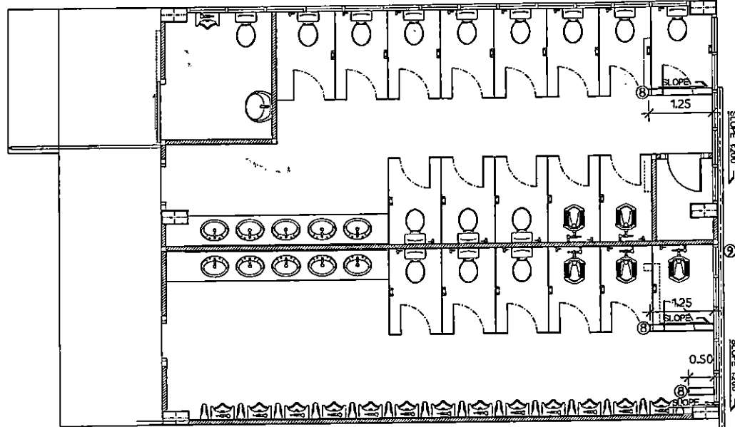
แปลนระบบระบายน้ำห้องน้ำได้ดูแลอาคารจกลณี (ปรับปรุง) 1 : 75
