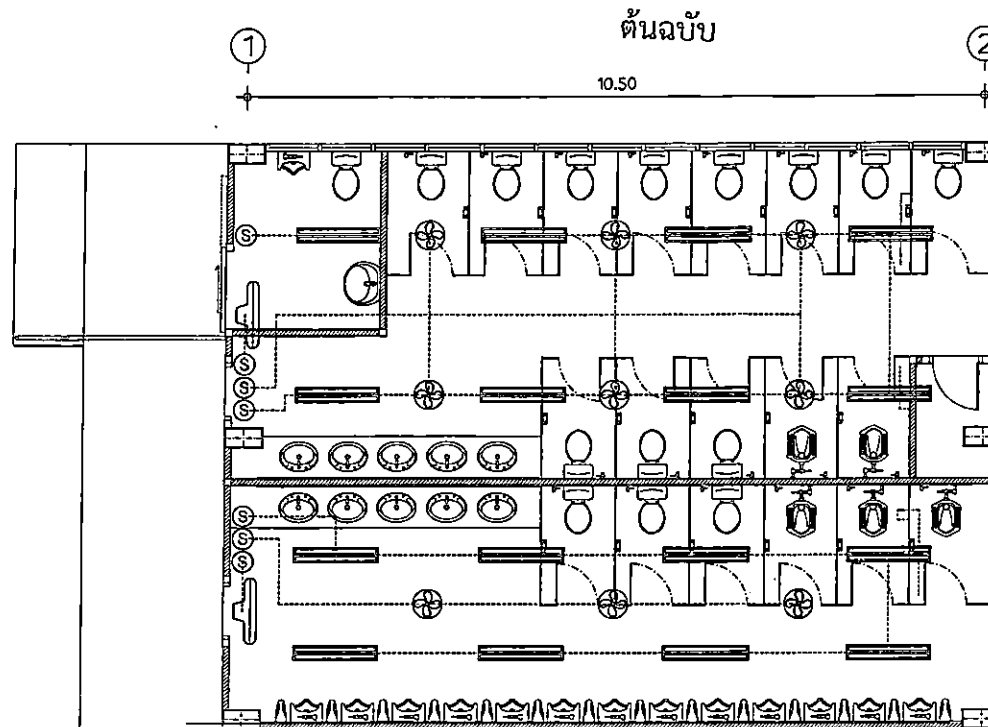
แปลนระบบไฟฟ้าห้องน้ำใต้ดินอาคารจกตณ (ปรับปรุง) 1 : 75
