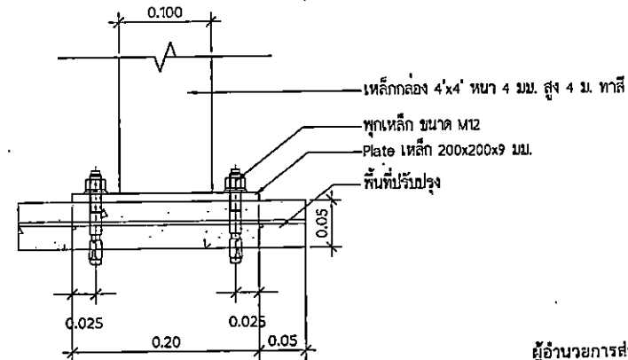
แบบขยายเสาด้านซ้ายหลัก
