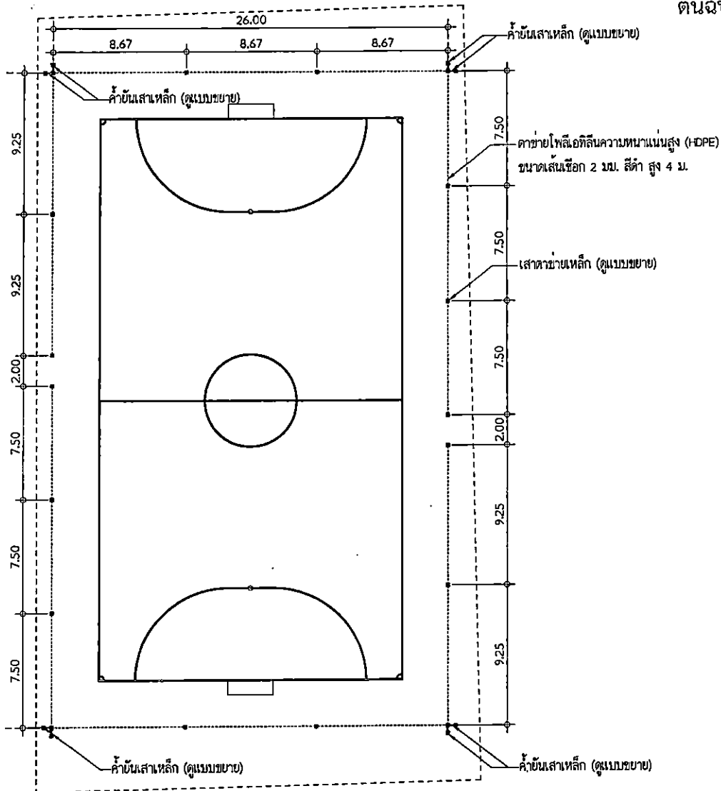
แปลงานตาข่ายกันลูกฟุตบอล 1 : 250
