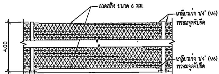
แปลงานตาข่ายกันลูกฟุตบอล 1 : 250
