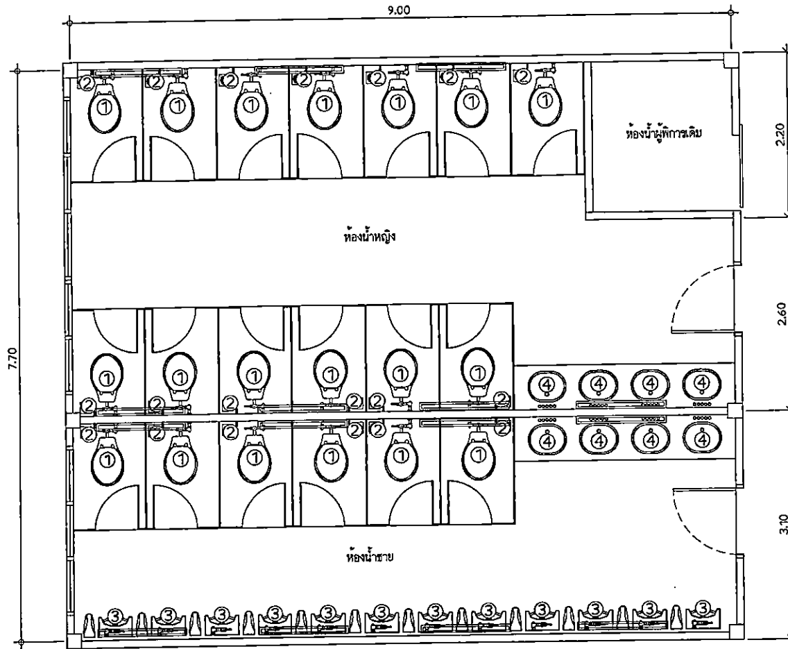
แปลนห้องน้ำร้านอาหาร เดิม (ปรับปรุง) 1 : 50
