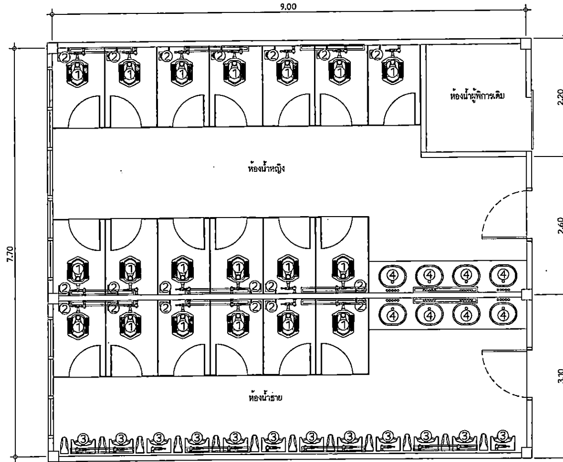
แปลนห้องน้ำโรงอาหาร เดิม (รื้อถอน) 1 : 50
