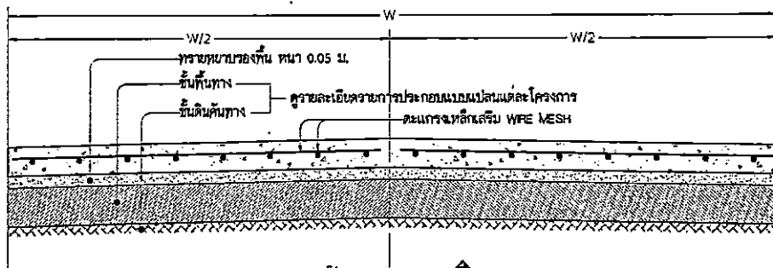
รูปตัด SCALE 1:25
