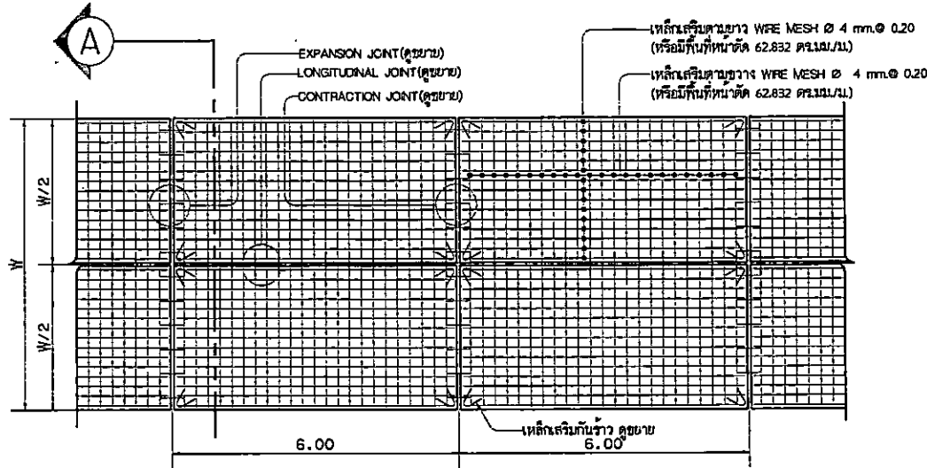
แปลนถนน ค.ส.ล. (หนา 0.15 ม.) SCALE 1:100
